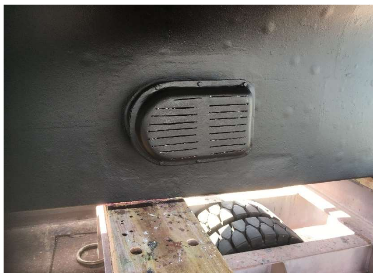
↓右舷側補機関吸い込み口
